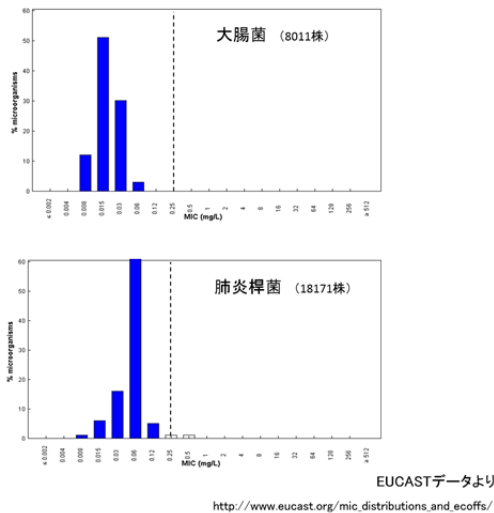
図1. 大腸菌および肺炎桿菌におけるメロペネムMIC分布 (EUCAST)
